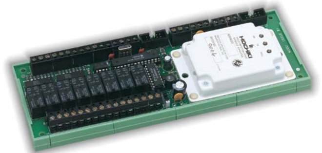
MIOU - Din rail mounting version (K559)
